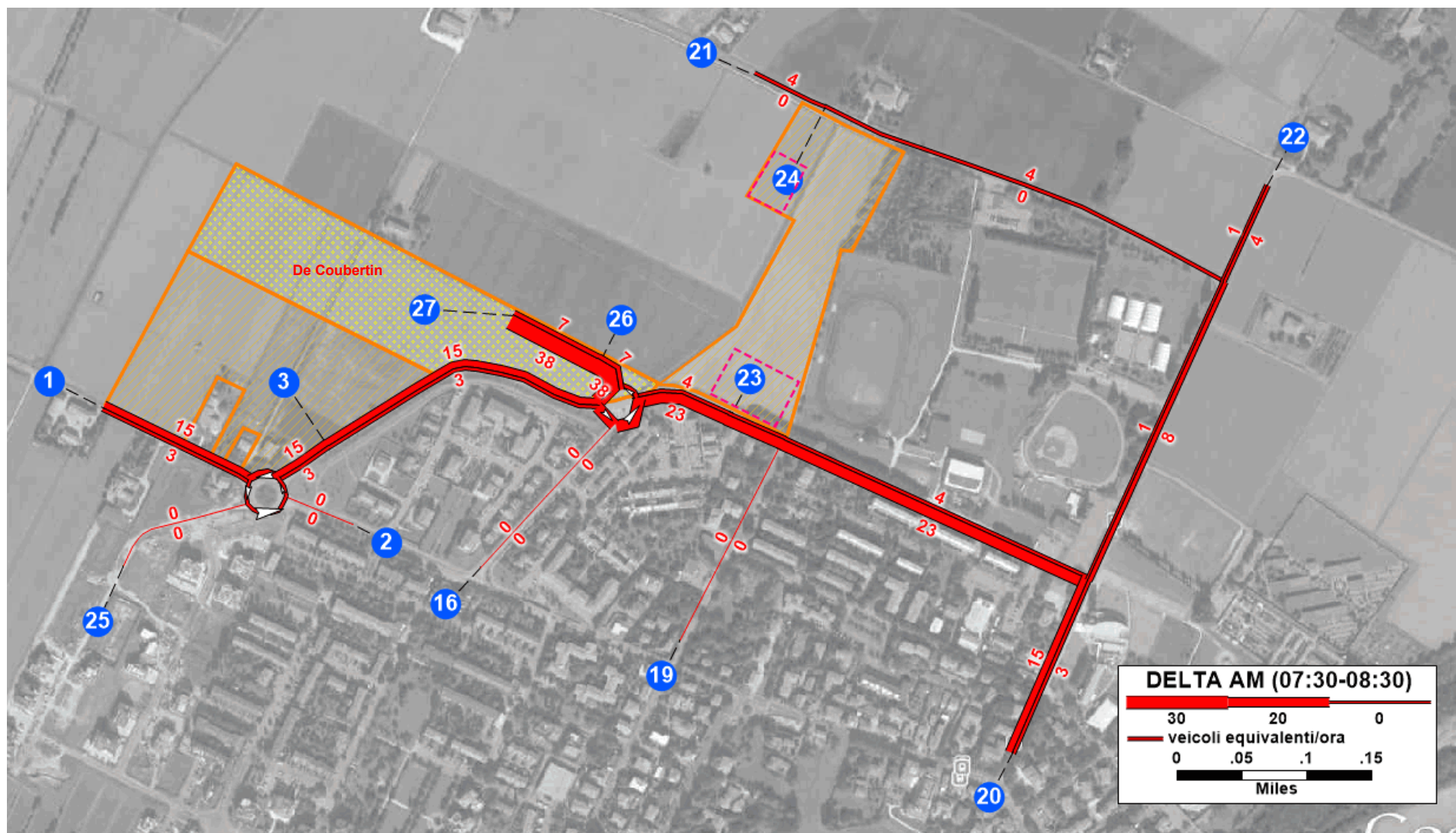
Figura 10- Flussogramma delta veicolare imputabile al sub-ambito "De Coubertin" (ora di punta AM)
