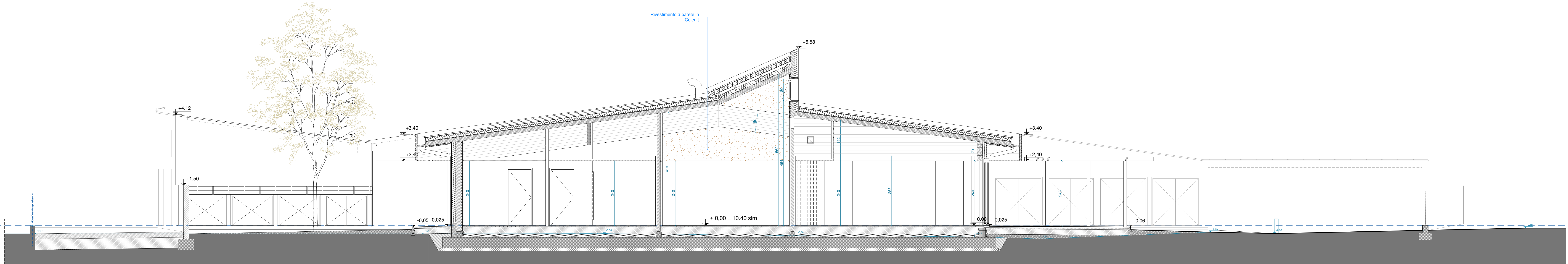
SEZIONE BB' Scala 1:50
