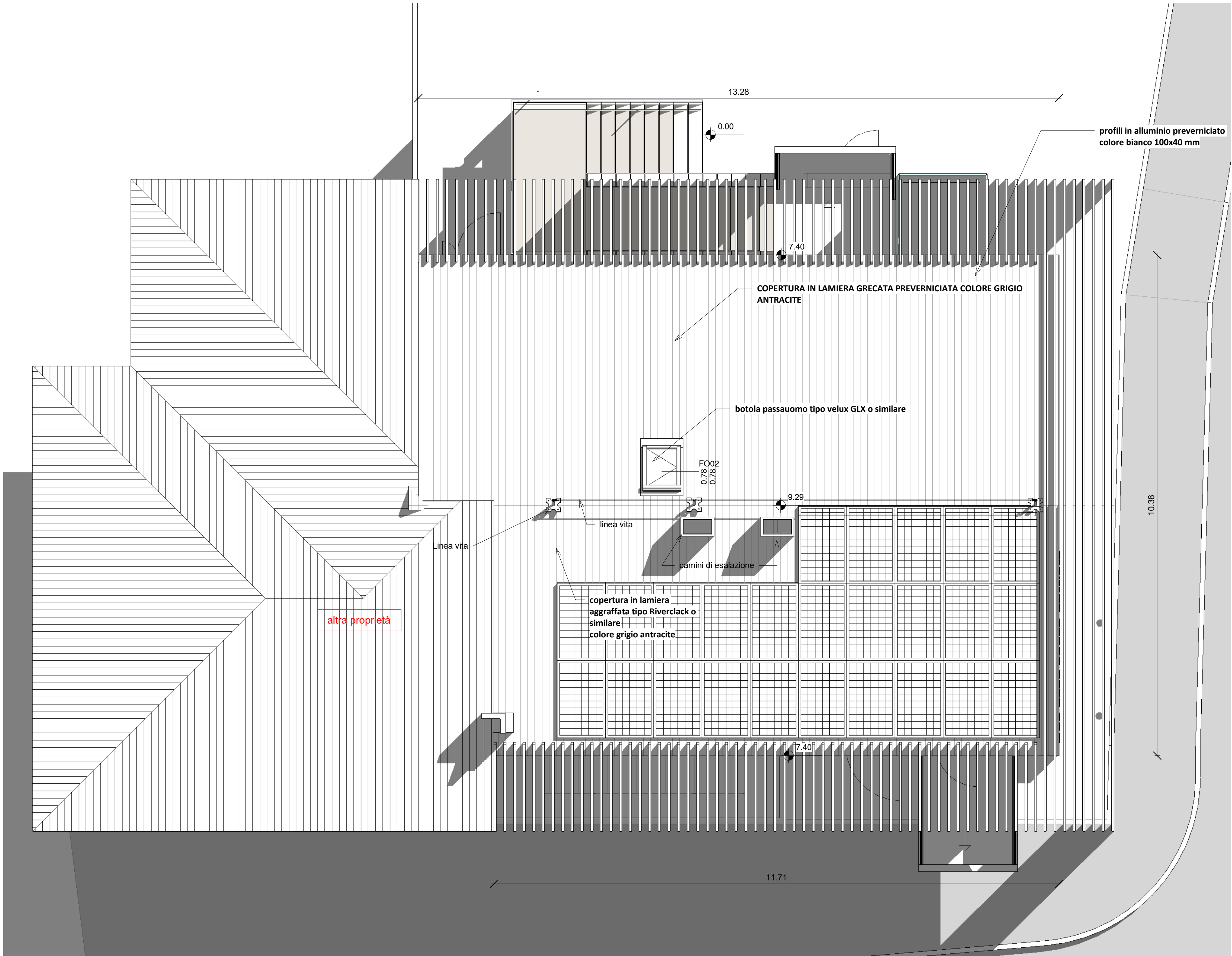
Colmo - VCO Scala 1 : 50
